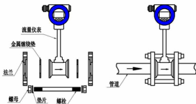
法兰卡装式的管道安装
